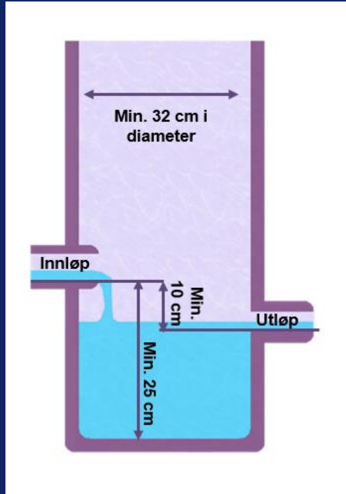
Anbefalt mål på prøvetakingskum
