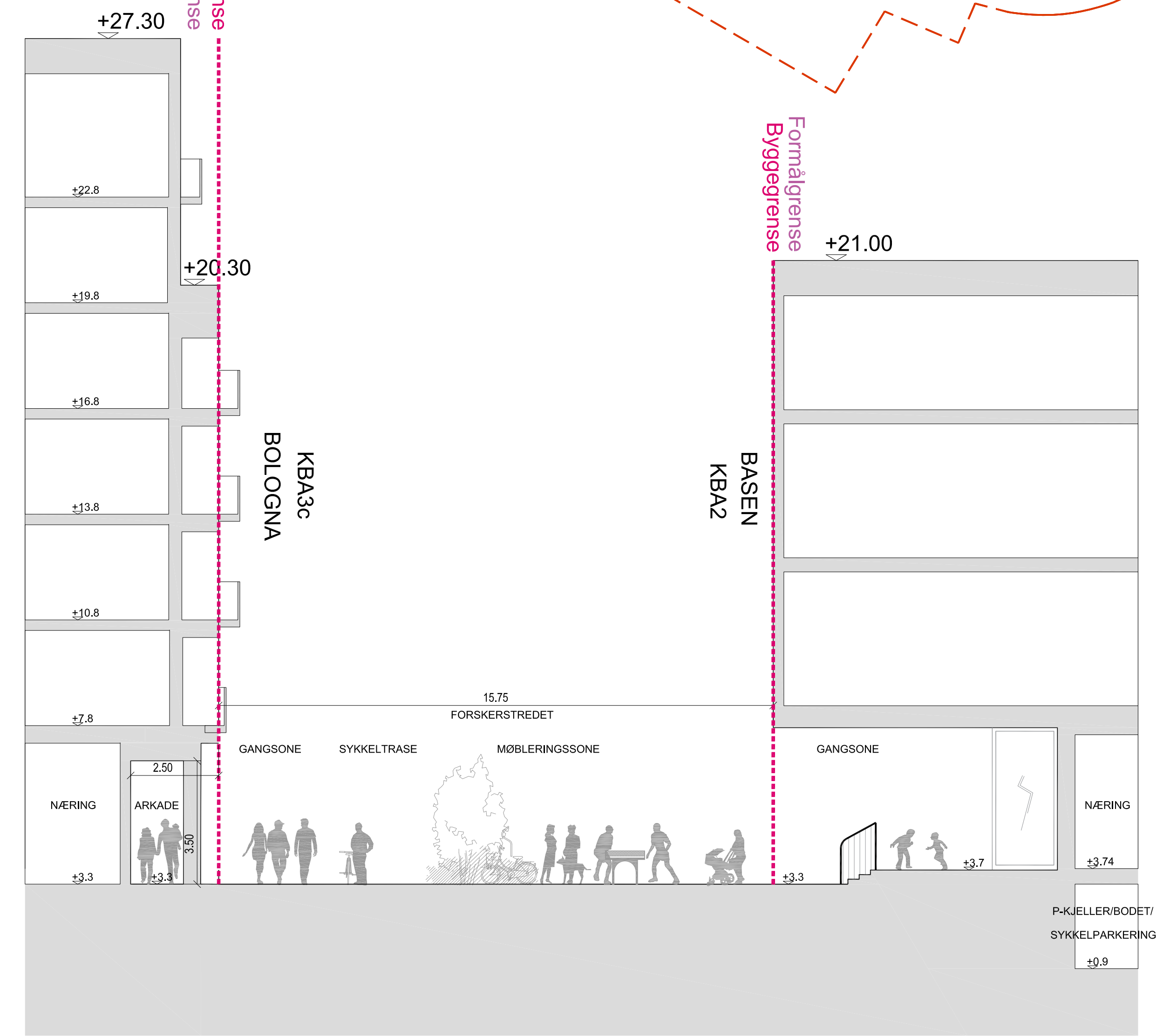
Snitt E-E'
