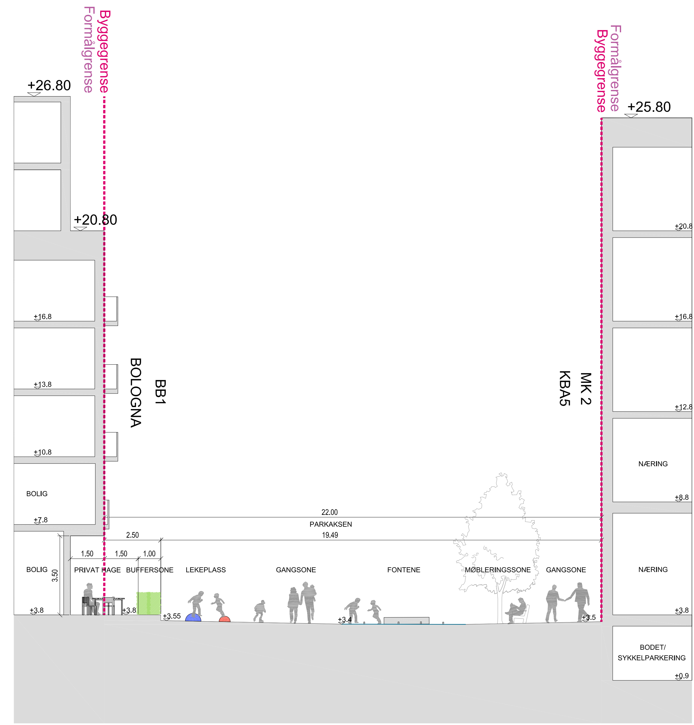
Snitt K-K'
