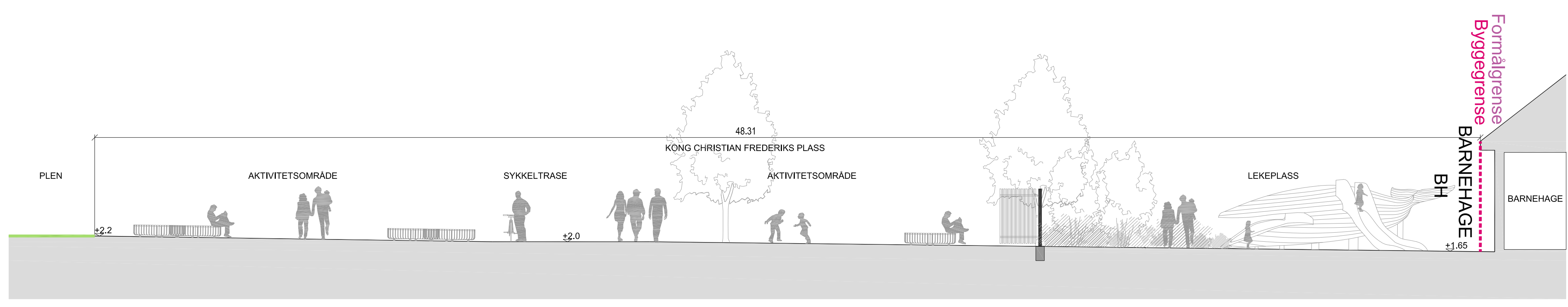
Snitt I-I'
