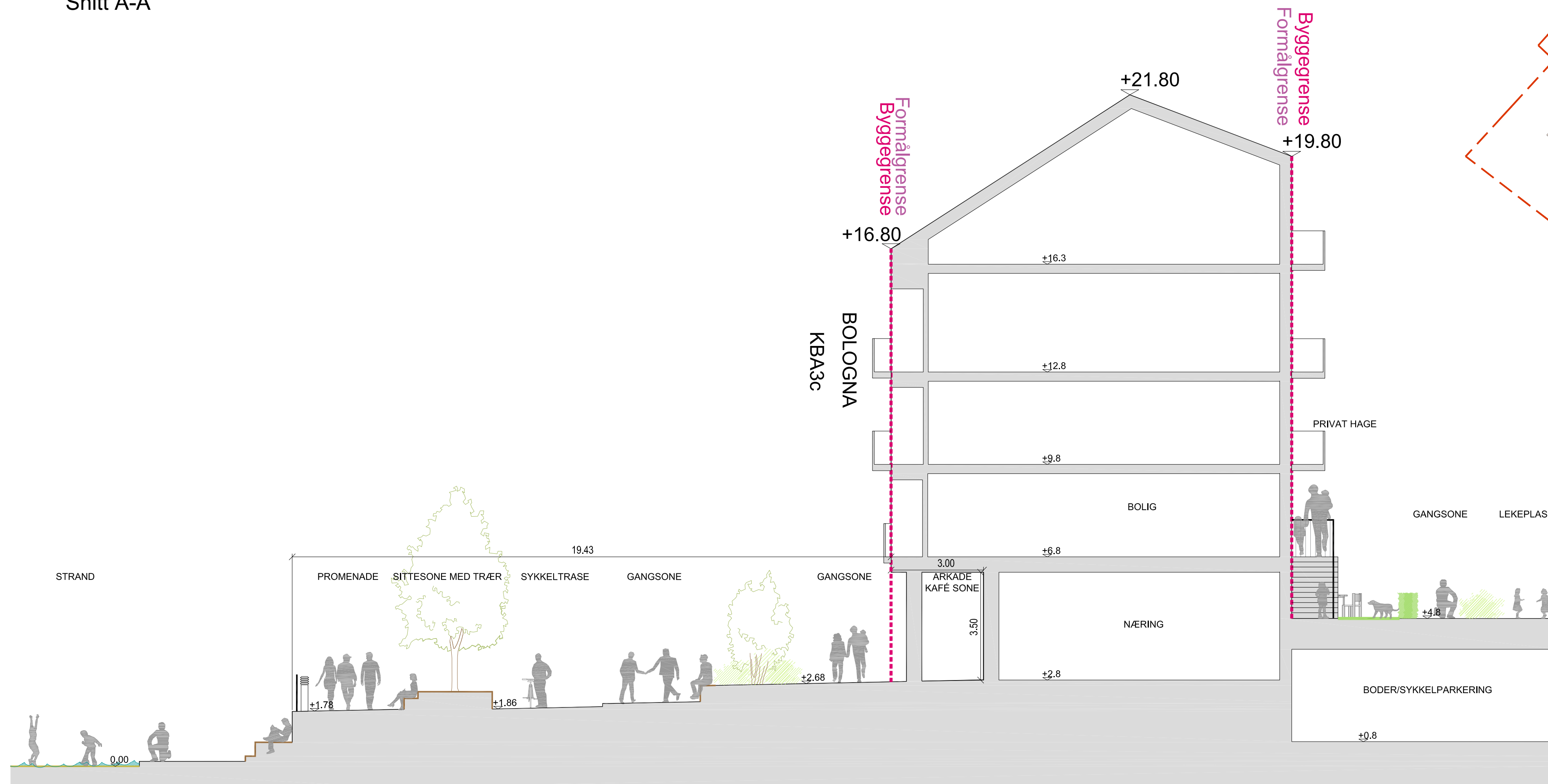
Snitt A-A'
