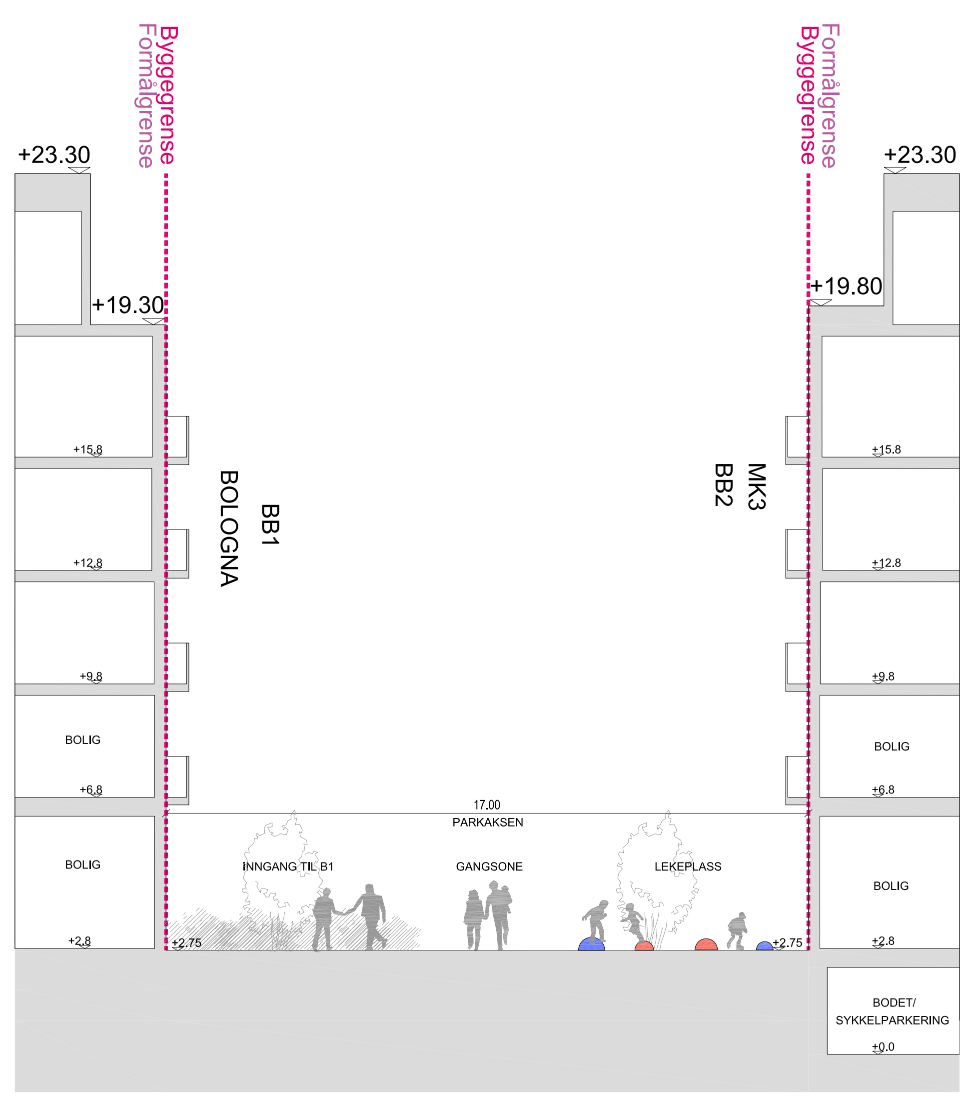
Snitt L-L'
