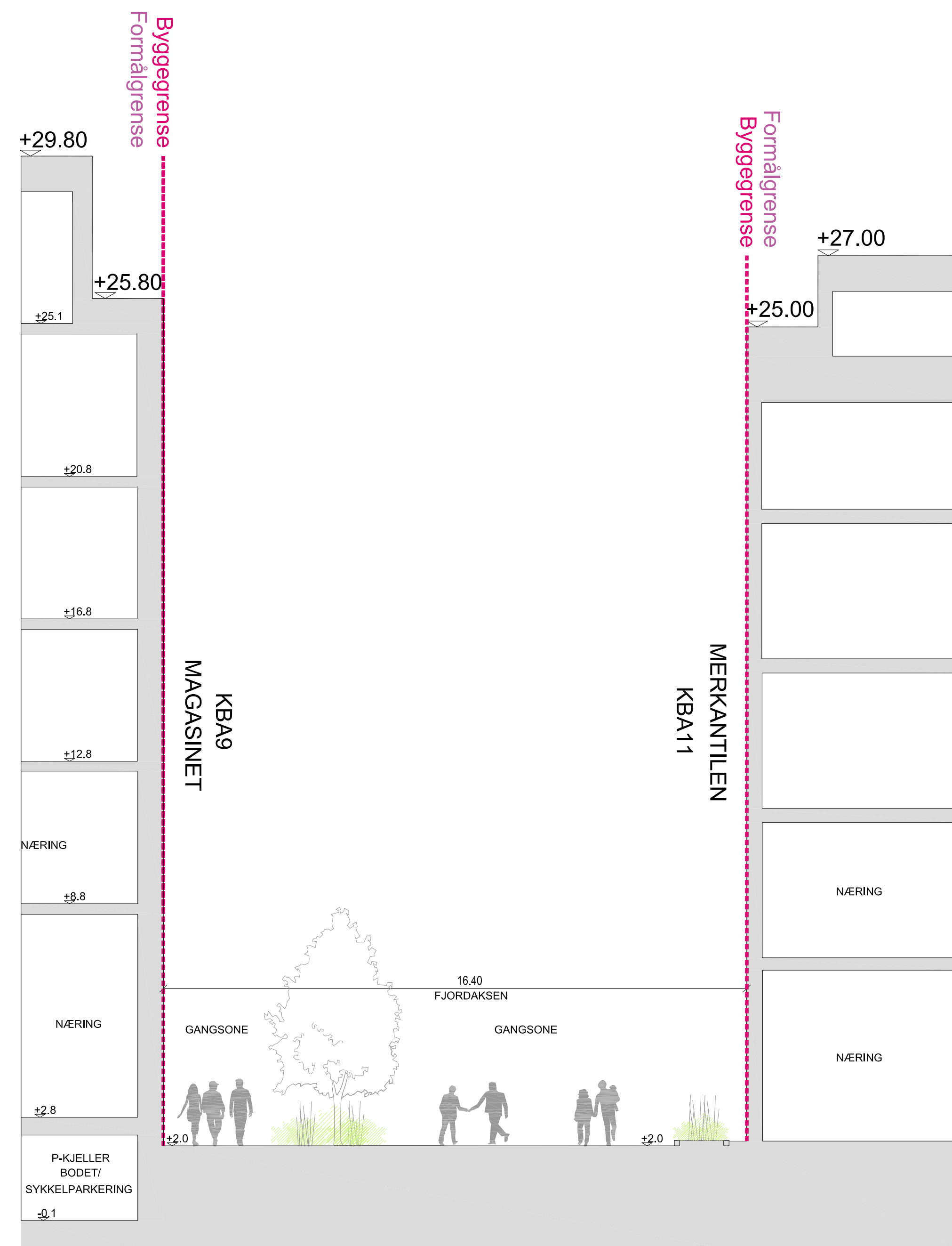
Snitt M-M'
