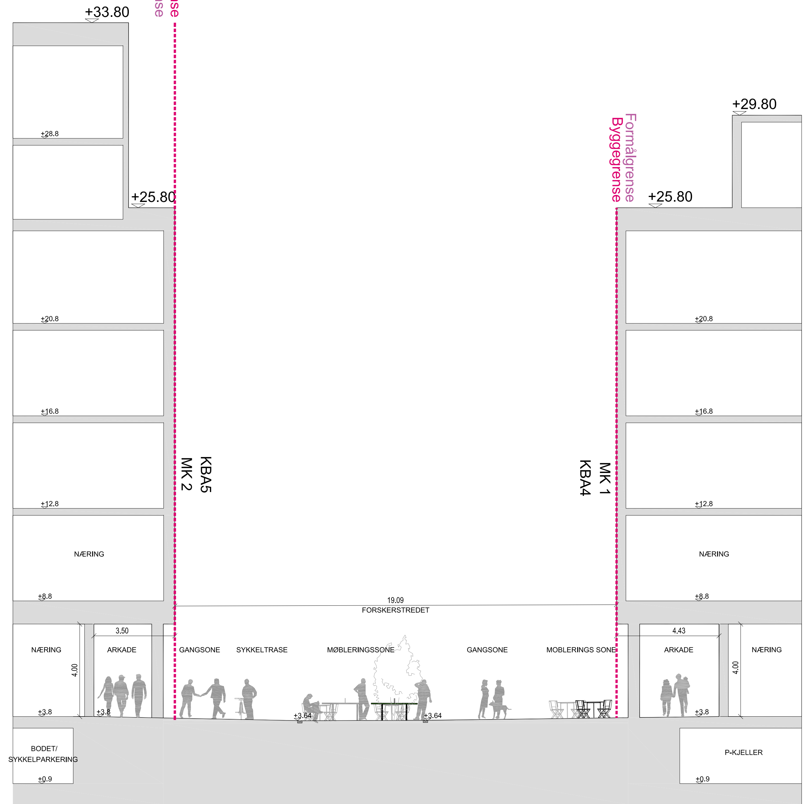
Snitt F-F'
