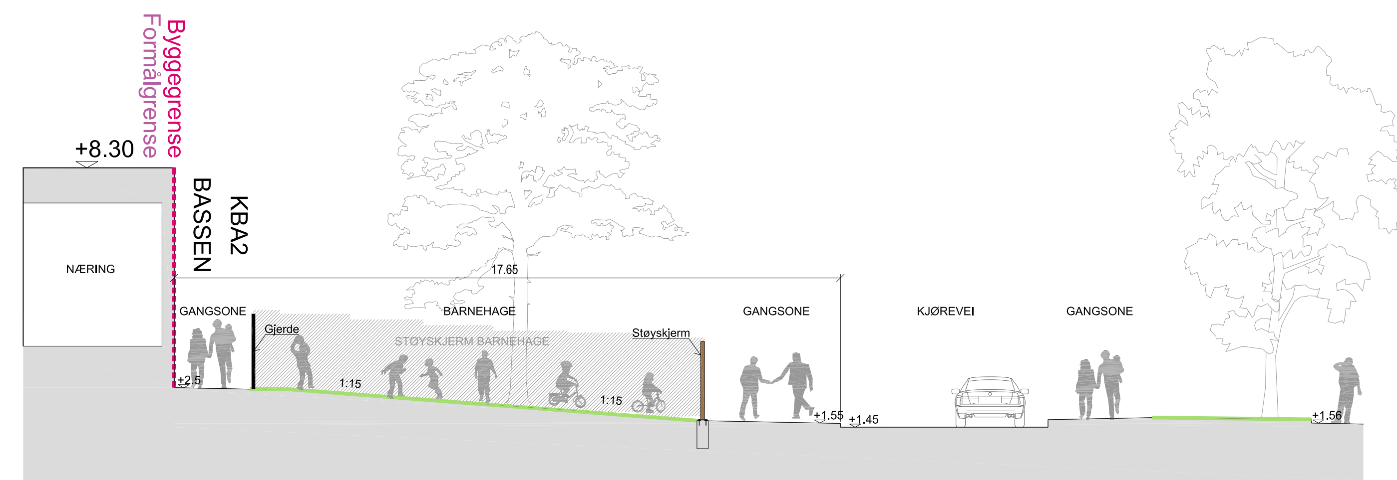
Snitt O-O'
