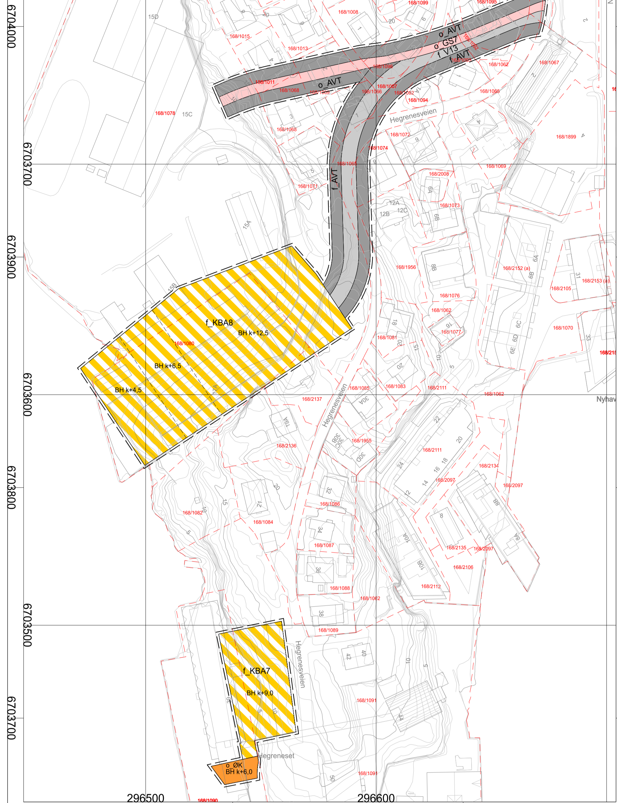
UTSNITT 3 - målestokk 1:1000 vertikalnivå 3 over grunnen
