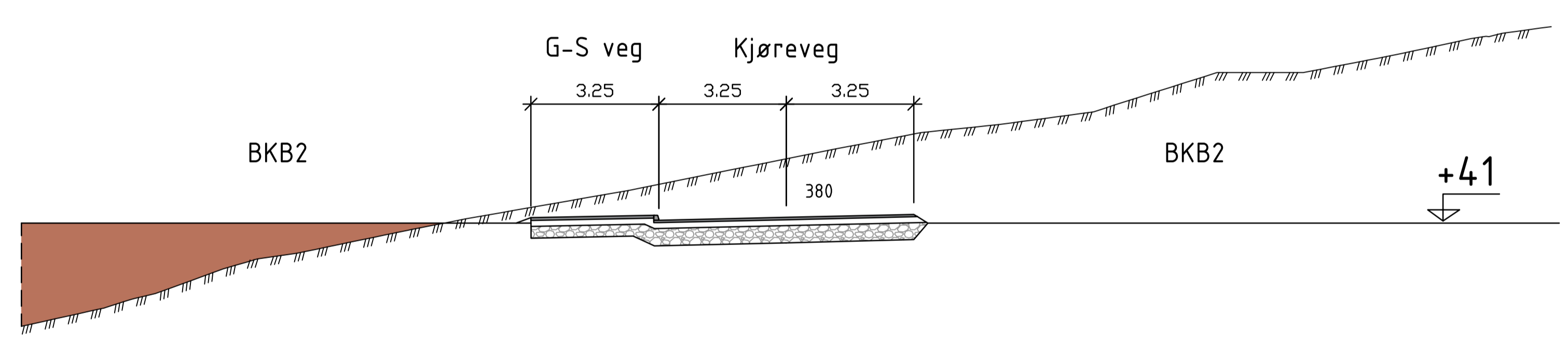
Snitt 5 Profil 380
