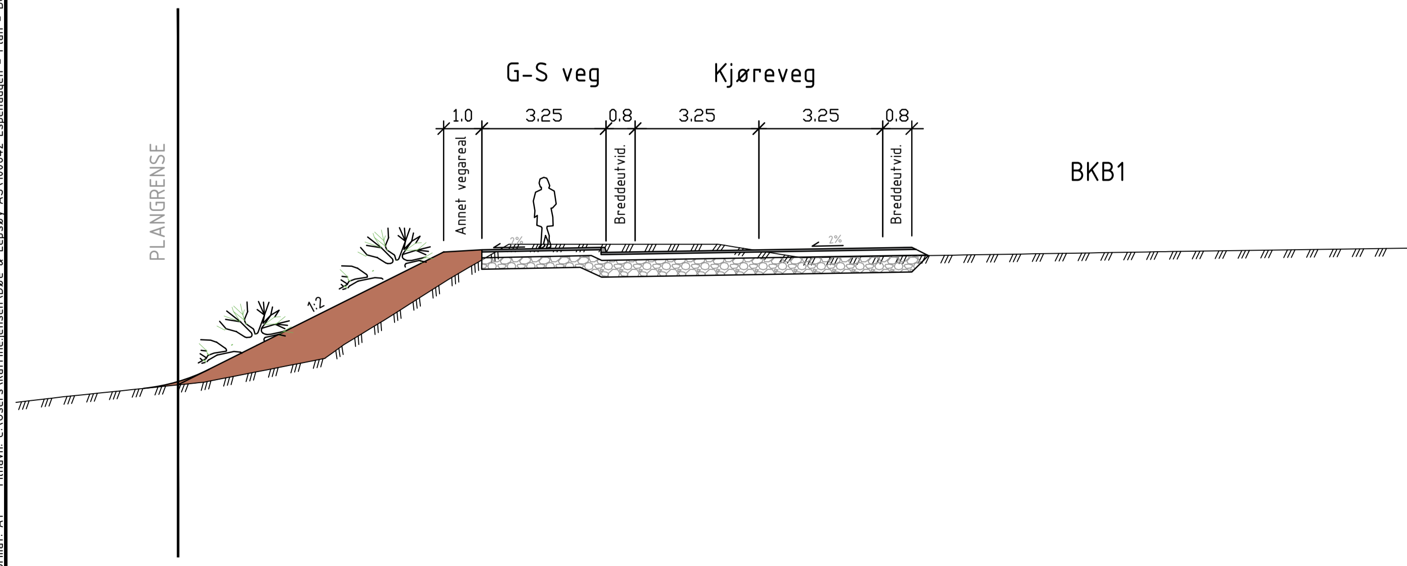
Snitt 3 Profil 320
