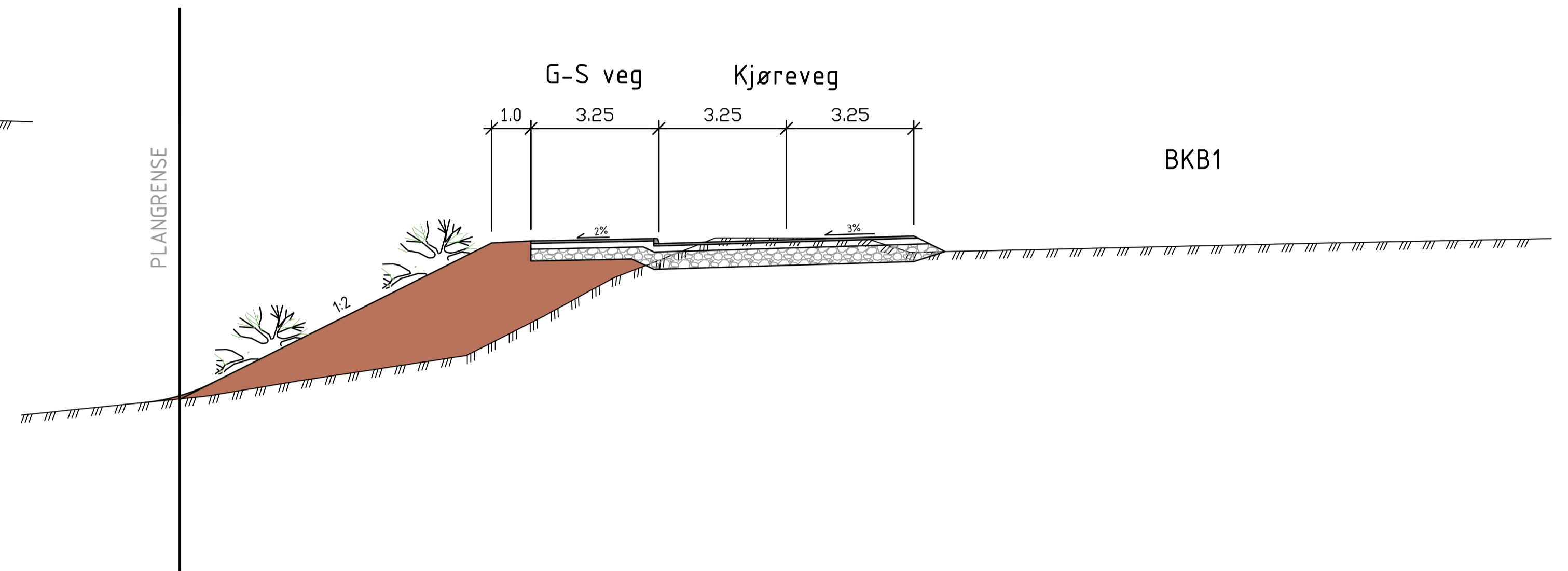
Snitt 5 Profil 380
