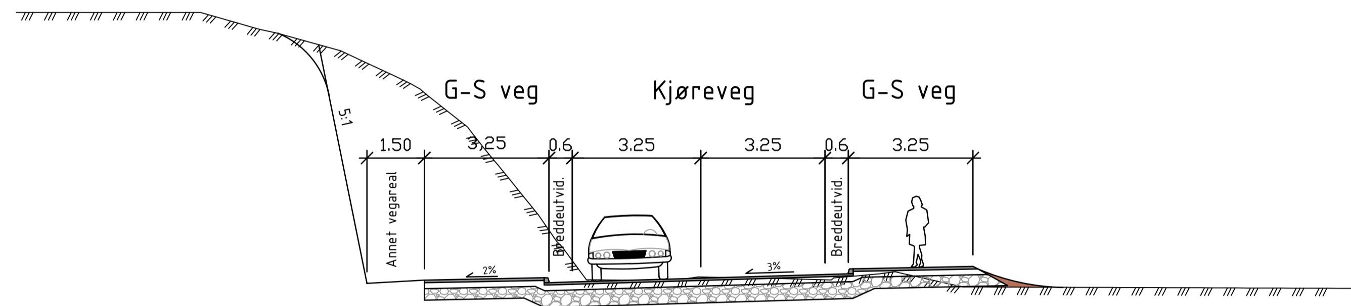
Snitt 2 Profil 230
