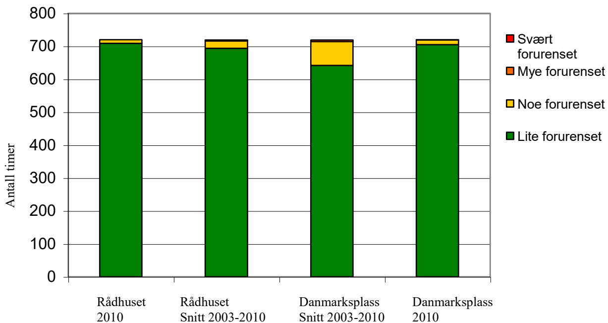
Luftkvalitet i april (antall timer fordelt etter helsevarsel)
